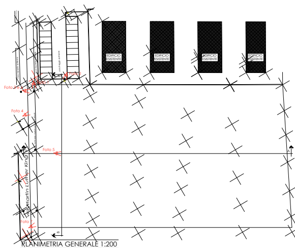
PLANIMETRIA GENERALE 1:200
